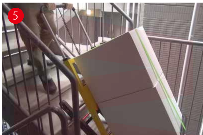
5 走行ベルト全体が階段に付くまで全体を倒します。
