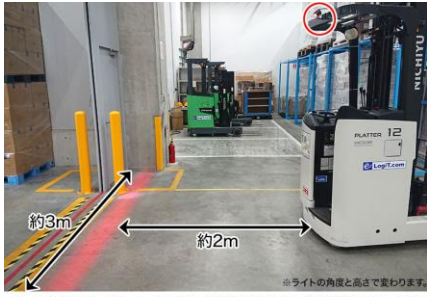
赤いLEDライトがフォークリフトの接近を知らせ、注意喚起を促します
